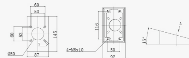
品名：15° 斜面
