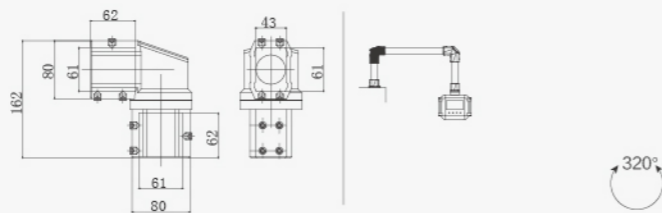
型号: JHY-ZJ2-4460-A
