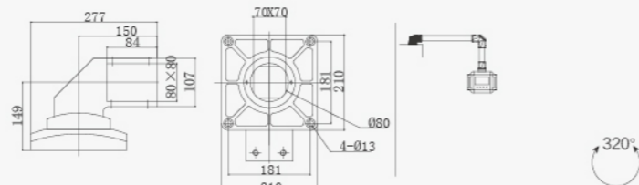
品名: 顶座
