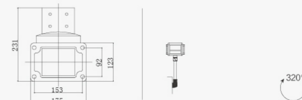
型号: JHY-QZ3-80
