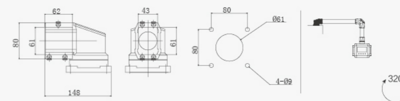
品名：顶座
