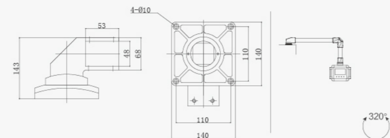
品名：顶座
