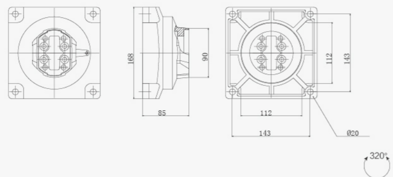
品名：墙座
